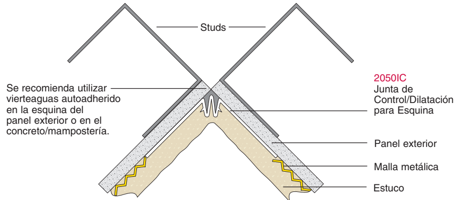
Junta de Control/Dilatación para Esquina Interior
